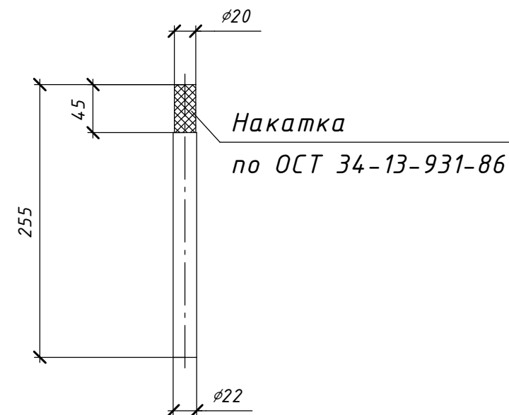
Поз. 4 (1:5)
