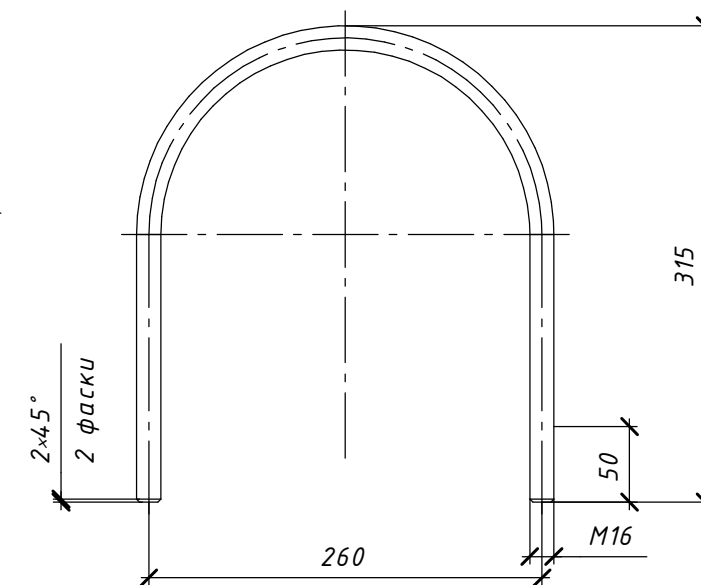
Поз. 5 (1:5)
