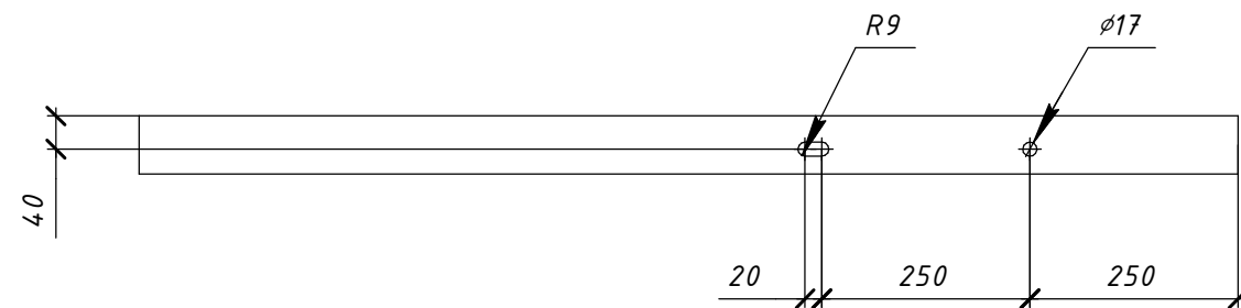
Поз. 1 (1:10)
